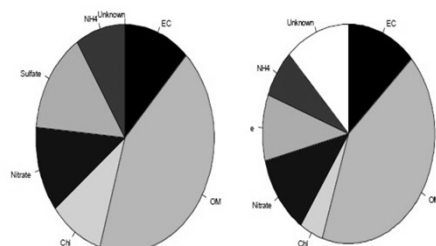
نتایج آنالیز شیمیایی PM2.5 هوای تهران ایستگاه تهرانسر - زمستان ۱۳۹۲
